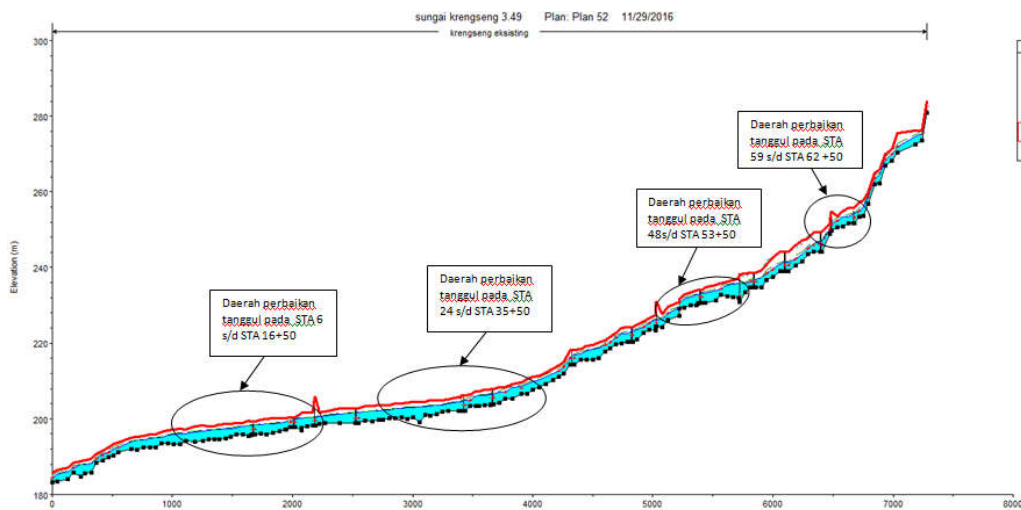
Gambar 7. Penampang Memanjang Sesudah Pendimensian Penampang Sungai
