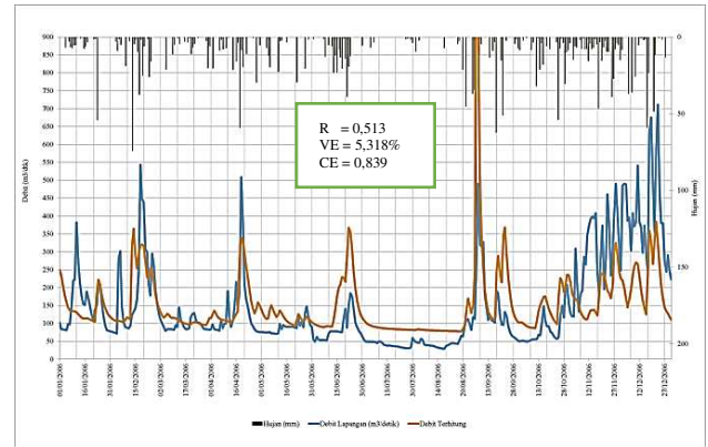
Gambar 12 Perbandingan Grafik Hidrograf Data Lapangan dari AWLR Dengan Data Terhitung Setelah Dikalibrasi Pada Curah Hujan Lapangan Tahun 2006
