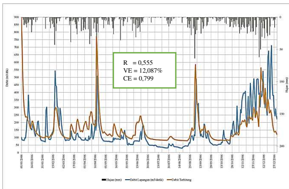
Gambar 15 Perbandingan Grafik Hidrograf Data Lapangan dari AWLR Dengan Data Terhitung Pada Curah Hujan Satelit Tahap Verifikasi Maju
