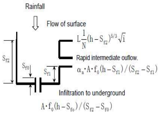
Gambar 2 Konsep Surface Model Sumber : Fukami, 2009
