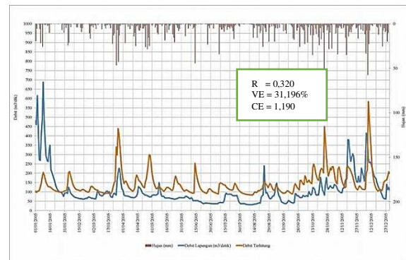
Gambar 5 Perbandingan Grafik Hidrograf Hasil Simulasi dengan Data Terukur dari AWLR Pada Kondisi Tanpa Kalibrasi untuk hujan satelit tahun 2005
