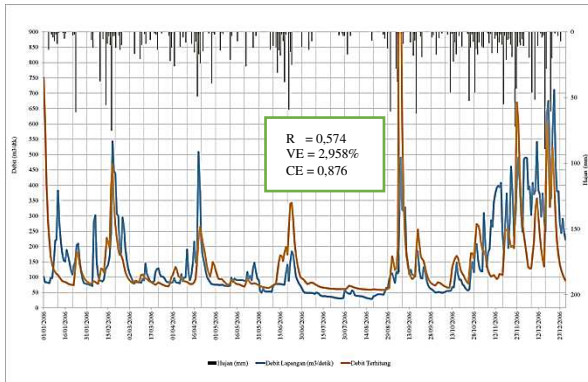
Gambar 10 Perbandingan Grafik Hidrograf Data Lapangan dari AWLR Dengan Data Terhitung Setelah Dikalibrasi Pada Curah Hujan Satelit Tahun 2006
