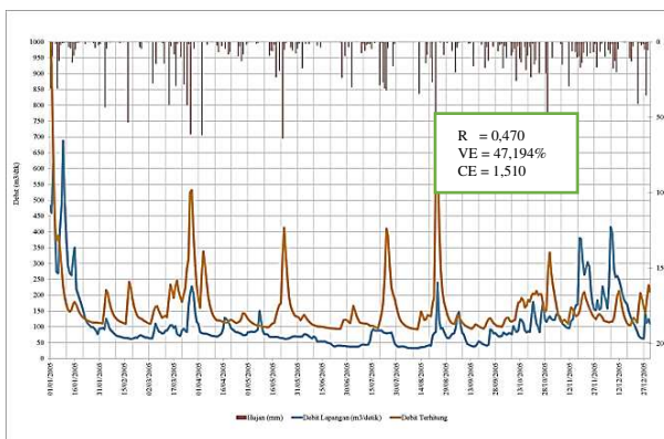
Gambar 11 Perbandingan Grafik Hidrograf Data Lapangan dari AWLR Dengan Data Terhitung Setelah Dikalibrasi Pada Curah Hujan Lapangan Tahun 2005
