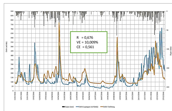
Gambar 6 Perbandingan Grafik Hidrograf Hasil Simulasi dengan Data Terukur dari AWLR Pada Kondisi Tanpa Kalibrasi untuk hujan satelit tahun 2006
