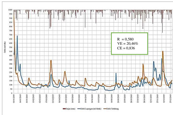
Gambar 13 Perbandingan Grafik Hidrograf Hasil Data Lapangan dari AWLR Dengan Data Terhitung Pada Hujan Modifikasi Tahap Kalibrasi pada Tahun 2005
