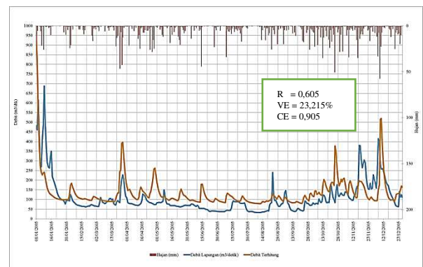
Gambar 9 Perbandingan Grafik Hidrograf Data Lapangan dari AWLR Dengan Data Terhitung Setelah Dikalibrasi Pada Curah Hujan Satelit Tahun 2005
