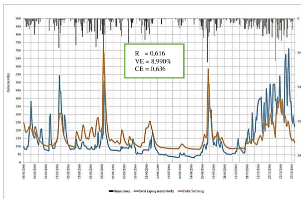
Gambar 14 Perbandingan Grafik Hidrograf Hasil Data Lapangan dari AWLR Dengan Data Terhitung Pada Hujan Modifikasi Tahap Kalibrasi pada Tahun 2006
