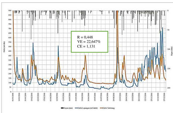
Gambar 16 Perbandingan Grafik Hidrograf Data Lapangan dari AWLR
