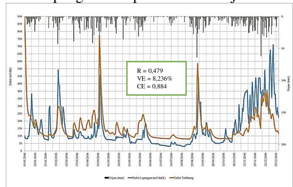
Gambar 17 Perbandingan Grafik Hidrograf Data Lapangan dari AWLR Dengan Data Terhitung Pada Curah Hujan Modifikasi Tahap Verifikasi Maju
