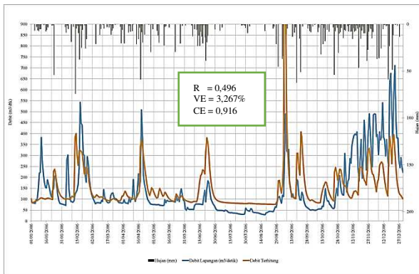
Gambar 8 Perbandingan Grafik Hidrograf Hasil Simulasi dengan Data Terukur dari AWLR Pada Kondisi Tanpa Kalibrasi untuk hujan lapangan tahun 2006
