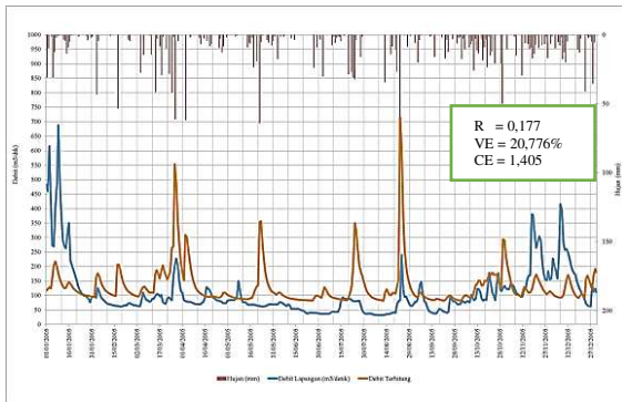
Gambar 7 Perbandingan Grafik Hidrograf Hasil Simulasi dengan Data Terukur dari AWLR Pada Kondisi Tanpa Kalibrasi untuk hujan lapangan tahun 2005
