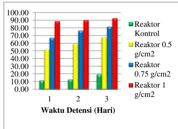
Gambar 3.1 Efisiensi Penyisihan COD Terhadap Kerapatan Tanaman pada Waktu Detensi
