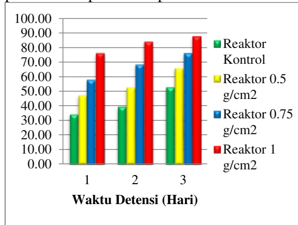
Gambar 3.2 Efisiensi Penyisihan TSS Terhadap Kerapatan Tanaman pada Waktu Detensi
