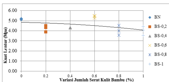
Gambar 11. Grafik kuat lentur beton
