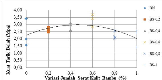
Gambar 10. Grafik kuat tarik belah beton
