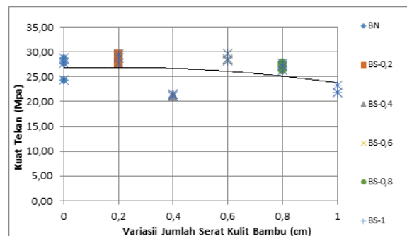
Gambar 9. Grafik kuat tekan beton
