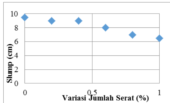
Gambar 8. Grafik slump beton
