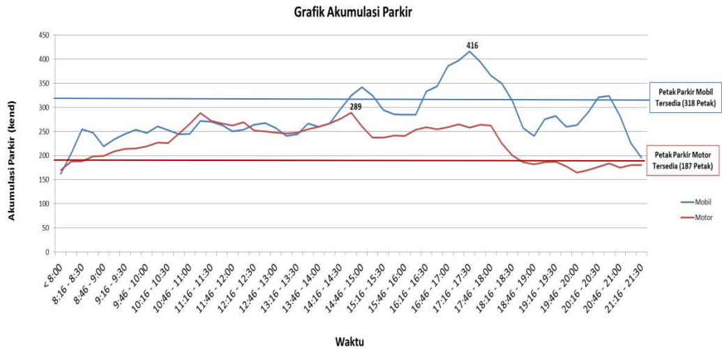
Gambar 2. Grafik Akumulasi Parkir Maksimum (Sabtu, 16 Februari 2013)
