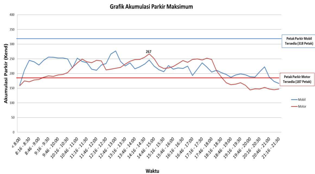
Gambar 1. Grafik Akumulasi Parkir Maksimum (Kamis, 14 Februari 2013)
