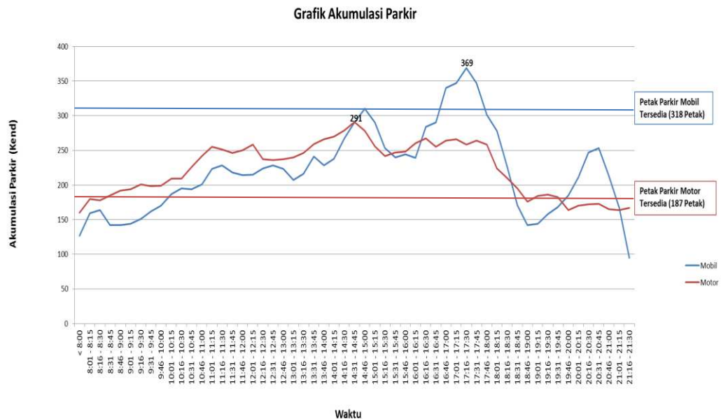
Gambar 3. Grafik Akumulasi Parkir Maksimum (Minggu, 17 Februari 2013)
