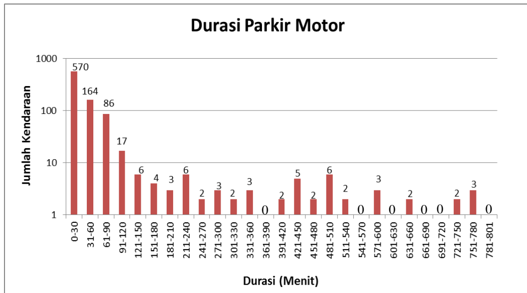
Gambar 5. Grafik Durasi Parkir Motor (Kamis, 14 Februari 2013)
