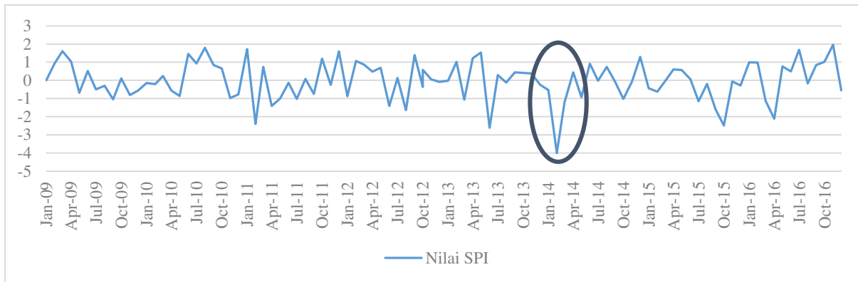
Grafik 1. Indeks Kekeringan pada Grid 21, Pulau Tebing Tinggi Tahun 2009 – 2016 Periode 1 Bulanan (Sumber: Hasil Perhitungan)
