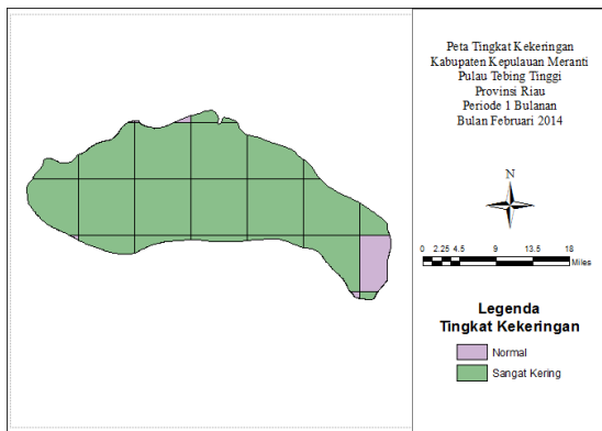
Gambar 5. Tingkat Kekeringan di Bulan Februari 2014 Periode 1 Bulanan (Normal dan Sangat Kering) (Sumber: Hasil Perhitungan)
