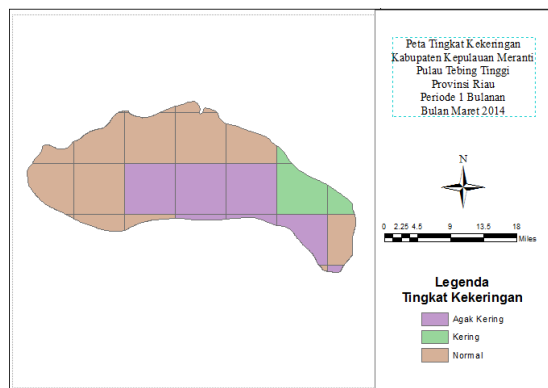
Gambar 6. Tingkat Kekeringan di Bulan Maret 2014 Periode 1 Bulanan (Agak Kering – Normal) (Sumber: Hasil Perhitungan)
