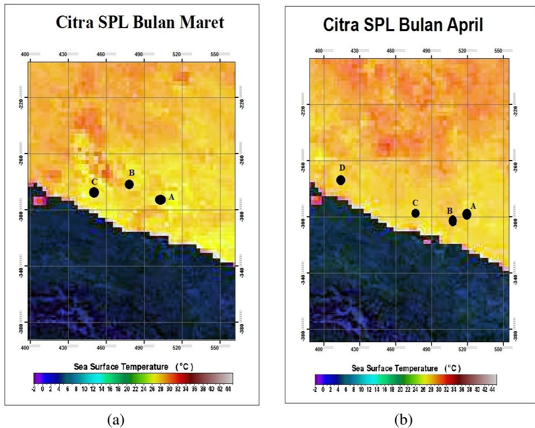
Gambar 2. (a) Citra SPL Maret, dan (b) Citra SPL April 2016.
