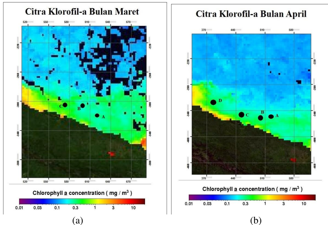
Gambar 3. (a) Citra klorofil-a Maret dan (b) Citra klorofil-a April 2016.
