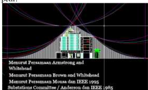
Gambar 6. Metode bola bergulir tampak Depan.
