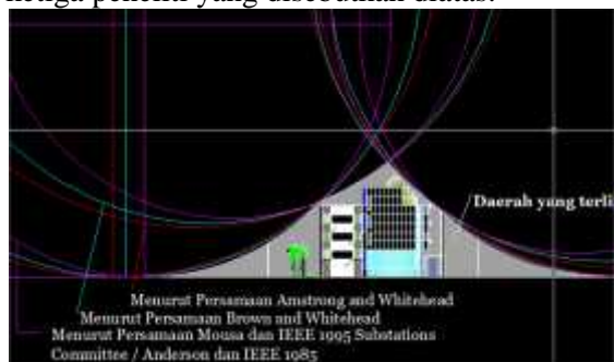
Gambar 5. Metode bola bergulir tampak belakang.
