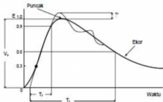
Gambar 1. Bentuk Tegangan impuls petir. Gambar 1. Bentuk tegangan impuls petir.
