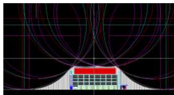
Gambar 8. Metode bola bergulir tampak samping kiri
