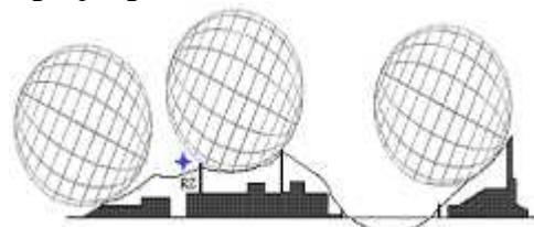
Gambar 3. Metode Bola Bergulir
