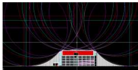
Gambar 7. Metode bola bergulir tampak samping kanan
