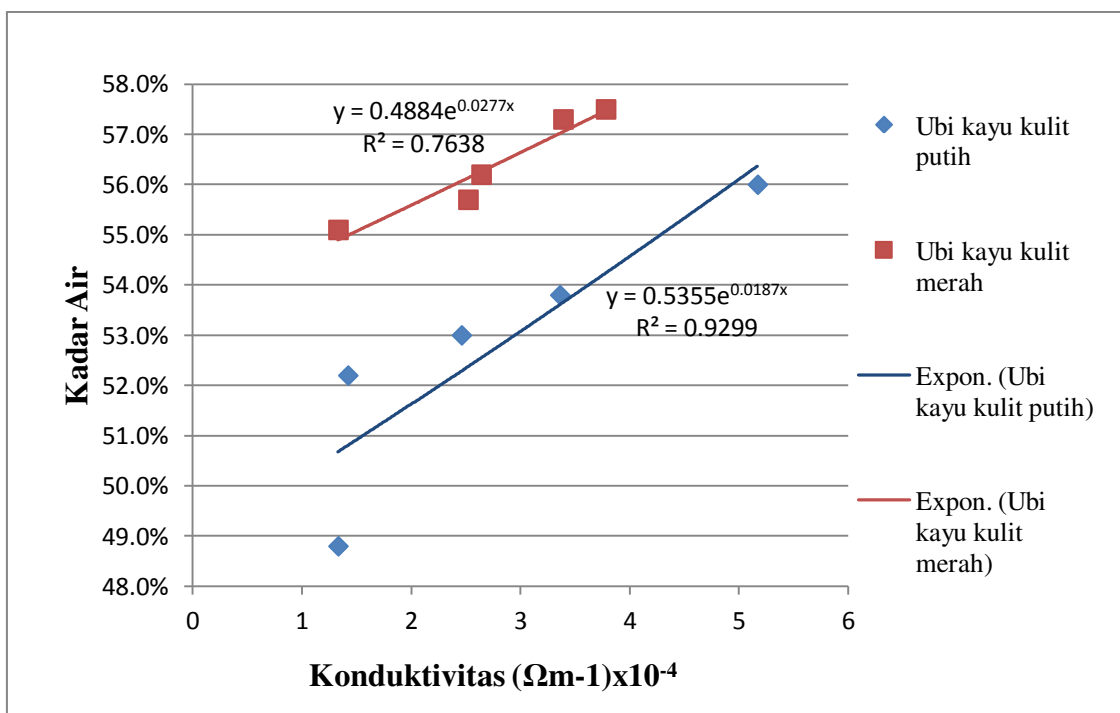
Gambar 4. Grafik hubungan antara konduktivitas terhadap kadar air ubi kayu putih dan ubi kayu kulit merah
