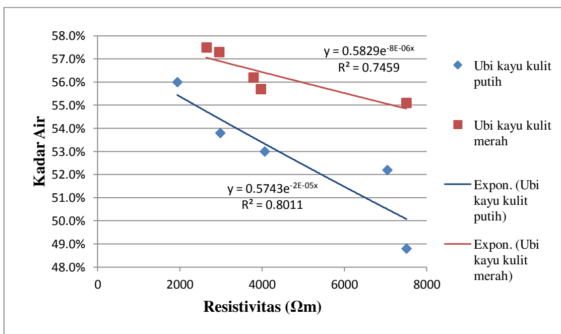
Gambar 3. Grafik hubungan antara resistivitas terhadap kadar air ubi kayu putih dan ubi kayu kulit merah
