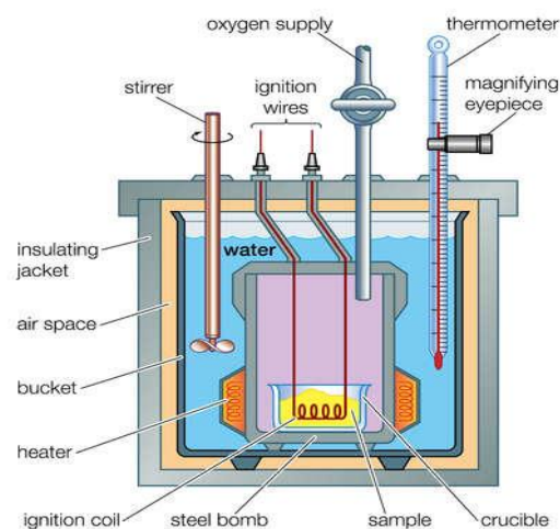
Gambar 1. Skema alat bom kalorimeter dalam kontainer (Mahajoeno, 2005)
