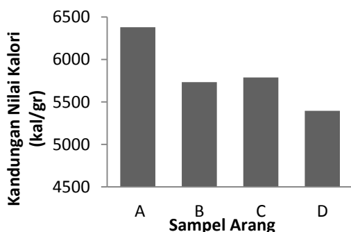
Gambar 2. Hubungan antara sampel arang setelah dicampur terhadap kandungan kalori rata- rata.
