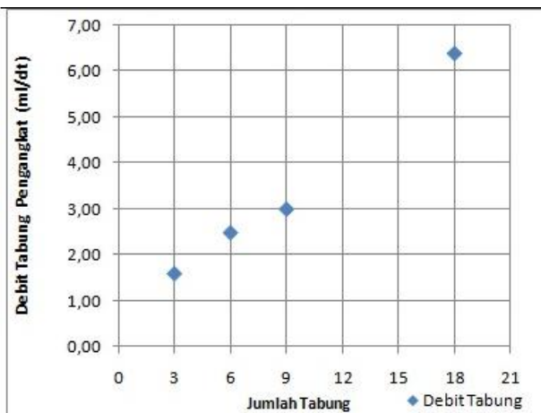
Gambar 5. Grafik jumlah tabung VS debit dari tabung (diameter 1,7 /tipe 3)
