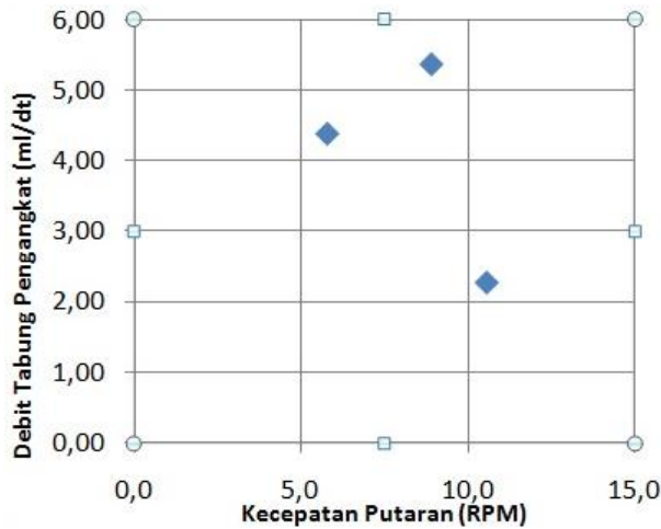
Gambar 8. Grafik jumlah putaran kincir dan debit dari tabung (diameter 1,7 / tipe 3)
