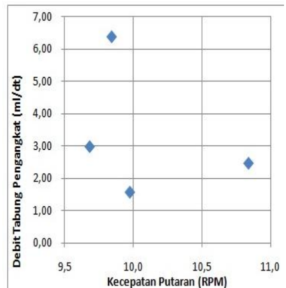
Gambar 7. Grafik jumlah putaran kincir dan debit dari tabung (diameter 1,3 / tipe 2)
