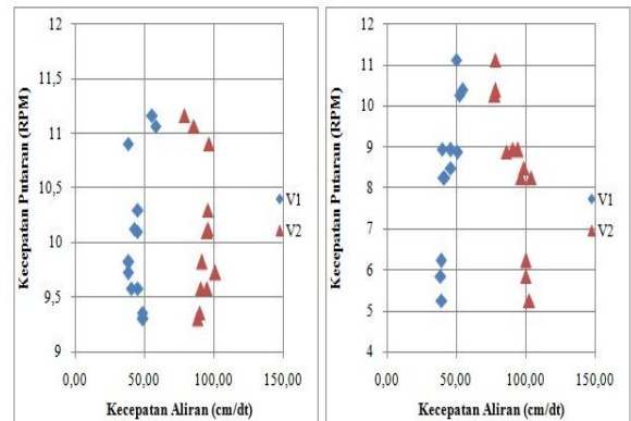
a. Diameter tabung 1,3 cm
