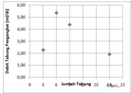
Gambar 6. Grafik jumlah tabung VS debit dari tabung (diameter 1,7 /tipe 3)
