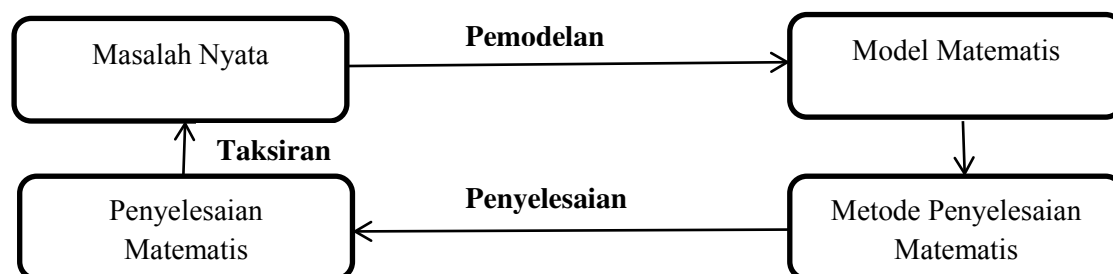
Gambar 4 Alur Penyelesaian Masalah Secara Matematik
