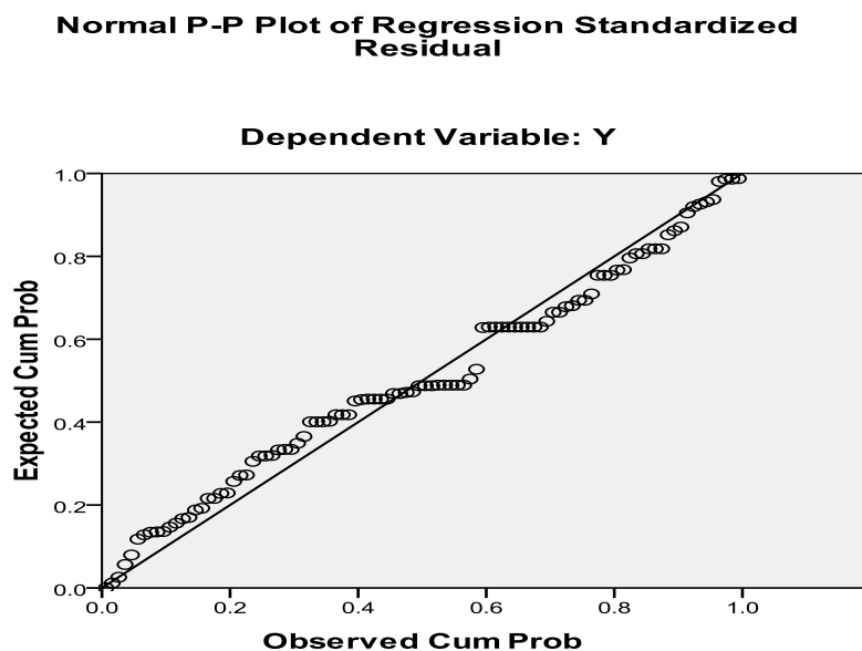
Gambar 3 Uji Normalitas
