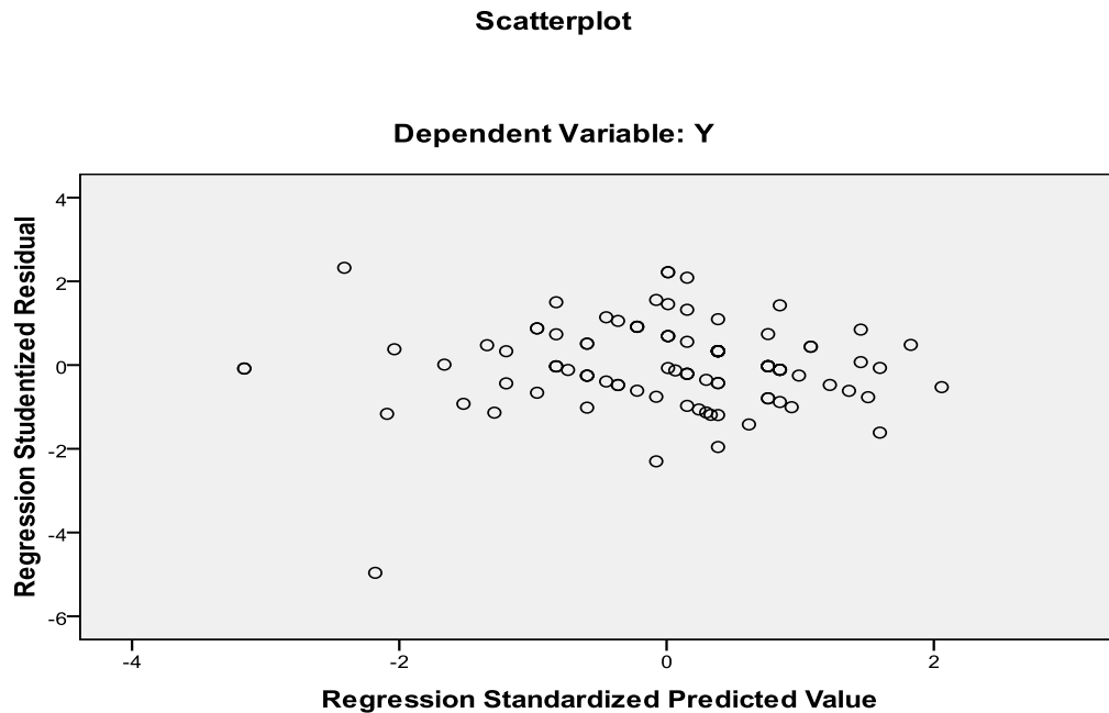
Gambar 2 Uji Heteroskedastisitas
