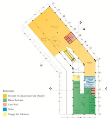
Gambar 24 Denah Lantai Dua
