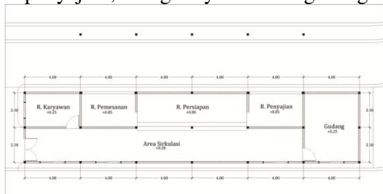
Gambar 30 Denah Fasilitas Drive Thru Sumber: Hasil Pengembangan Desain, 2015
