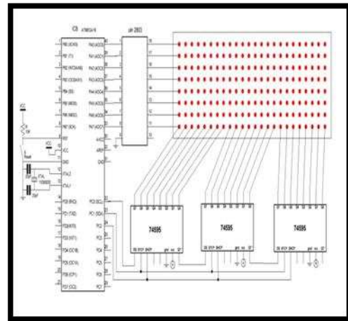
Gambar 7 Rangkaian Dotmatrik
