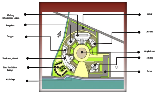
Gambar 9. Tatanan Massa
