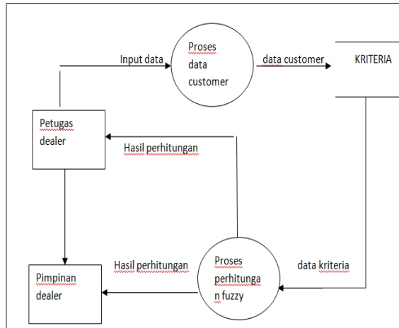
Gambar 4 Dfd Level 1
