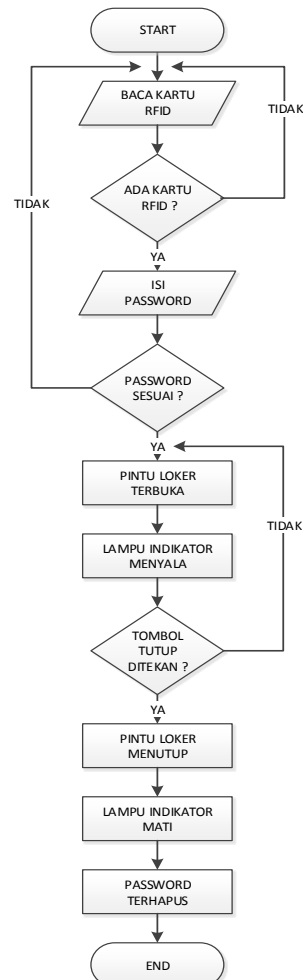
Gambar 3. 4 Flowchart Proses Pengambilan Barang Dari Dalam Loker
