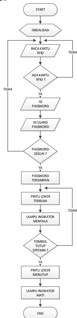
Gambar 3.3 Flowchart Proses Memasukkan Barang Ke Dalam Loker
