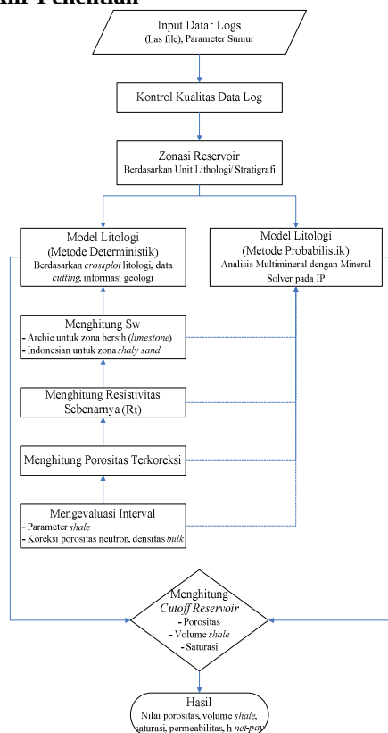
Gambar 3. Diagram Alir Analisis Petrofisika
