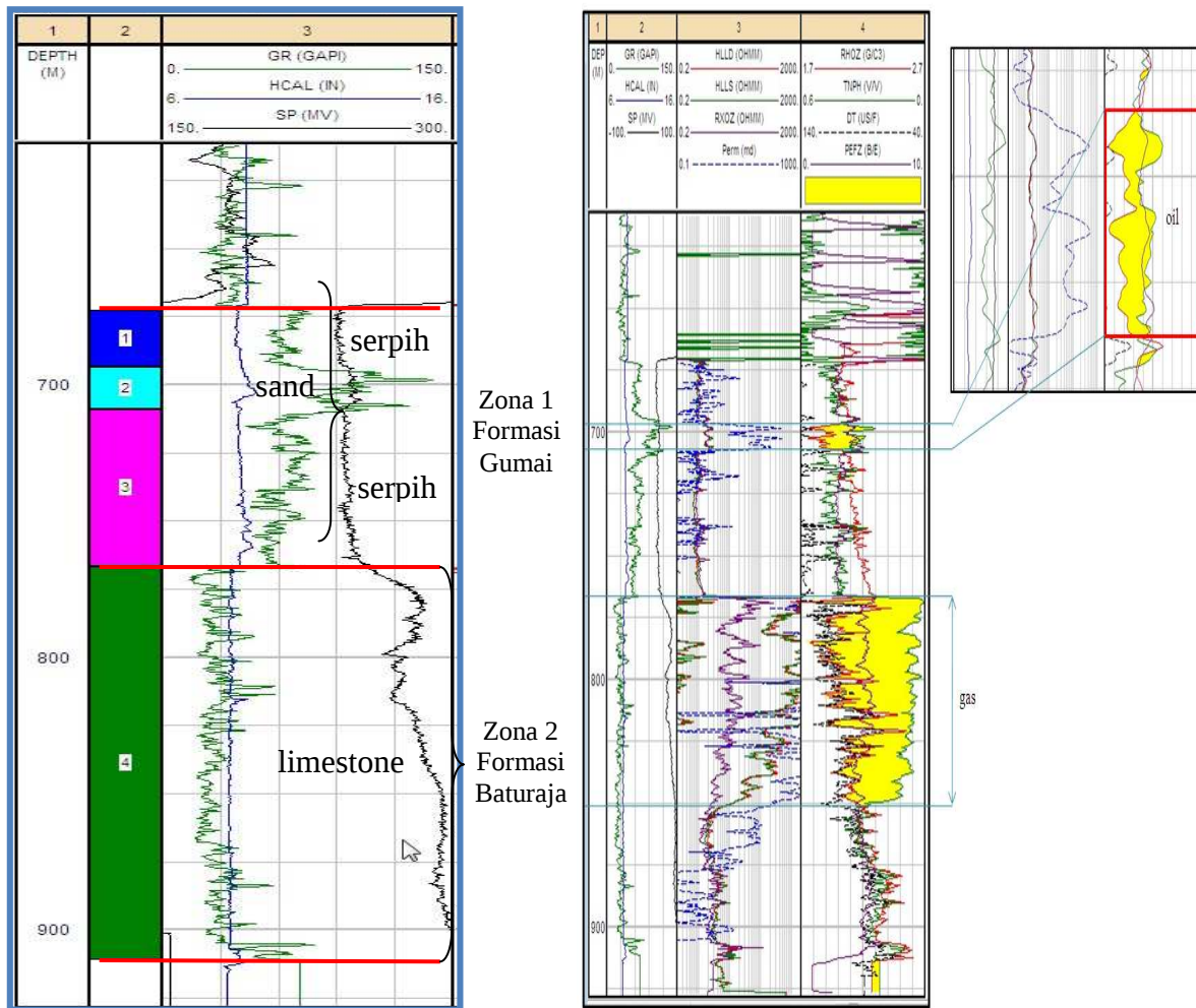
Gambar 5. Analisis Kualitatif untuk Membedakan Lapisan Batuan, Zonasi dan Fluida.
