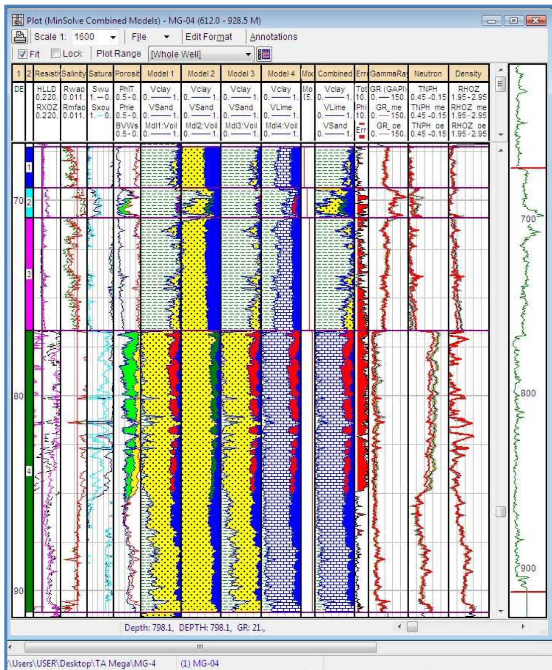
Gambar 13. Log Plot Hasil Analisis dengan Metode Probabilistik.
