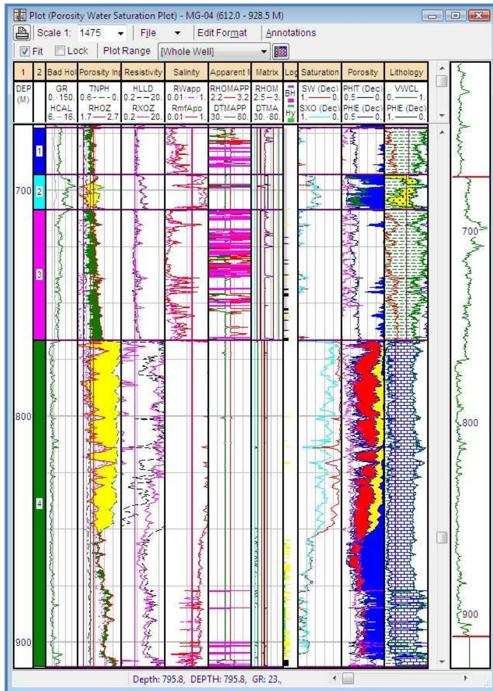
Gambar 6. Log Plot Hasil Analisis dengan Metode Deterministik.
