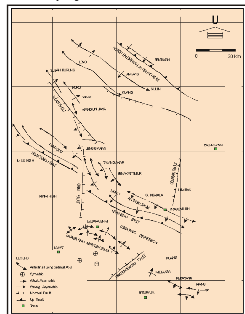
Gambar 2. Elemen Tektonik Regional Cekungan Sumatera Selatan (Pertamina, 2012)
