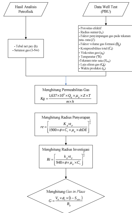
Gambar 4. Diagram Alir Perhitungan IGIP dengan well-basis
