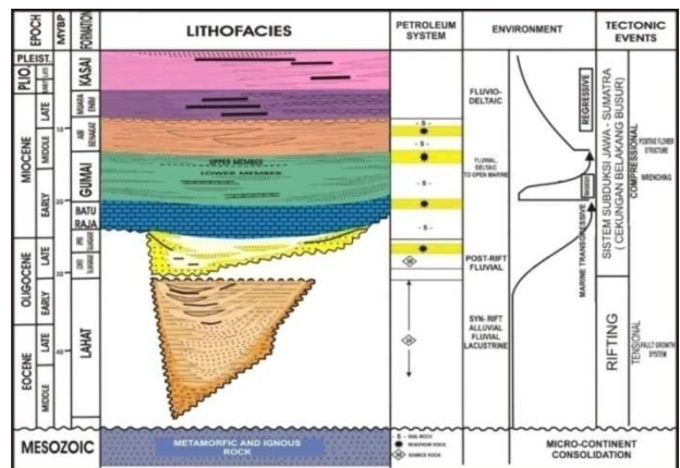
Gambar 1. Kolom Stratigrafi Cekungan Sumatera Selatan (sumber: Pertamina, 2012)
