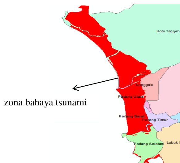
Gambar 1. Peta Kota Padang dan Zona Bahaya Tsunami
