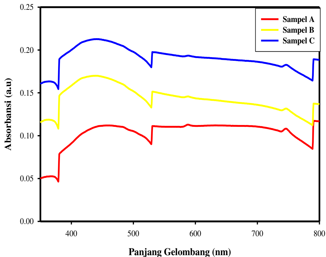
Gambar 2. Spektrum absorbansi dengan suhu 500 0 C pada sampel A, B, dan C
