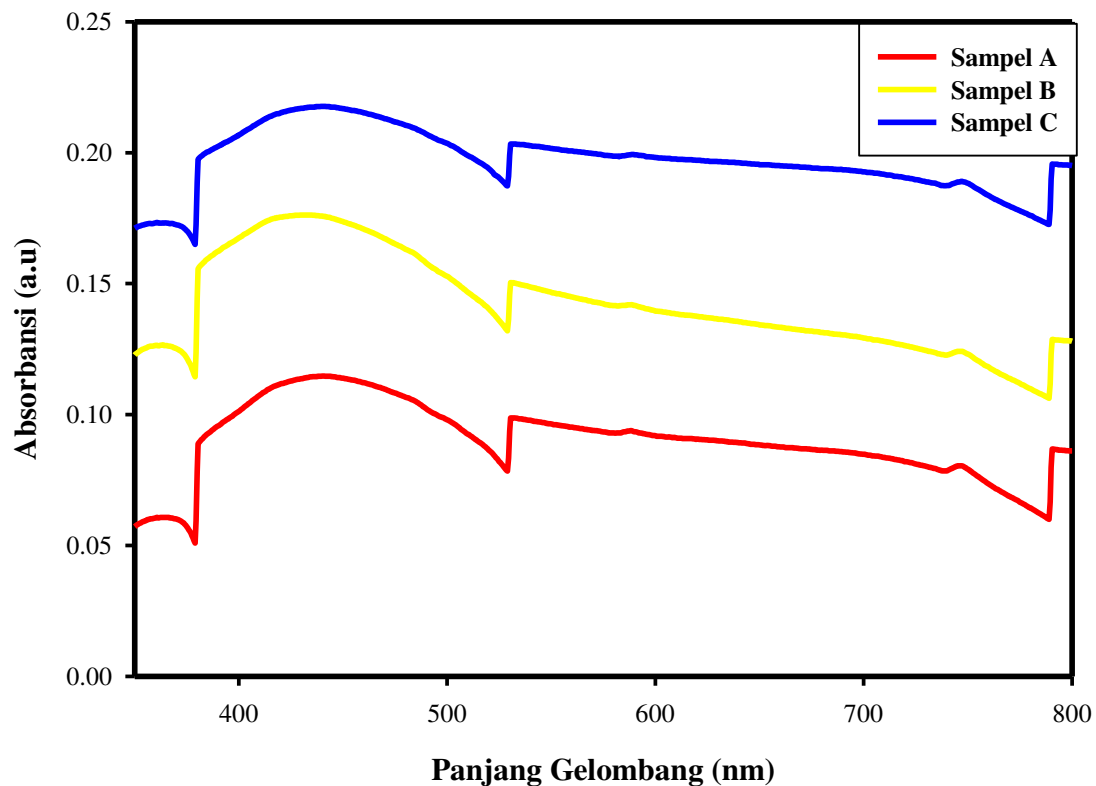
Gambar 3. Spektrum absorbansi dengan suhu 550 0 C pada sampel A,B dan C
