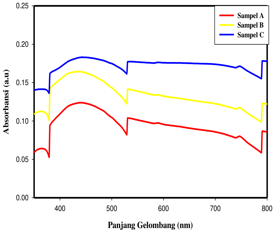
Gambar 4. Spektrum absorbansi dengan suhu 600 °C pada sampel A, B, dan C
