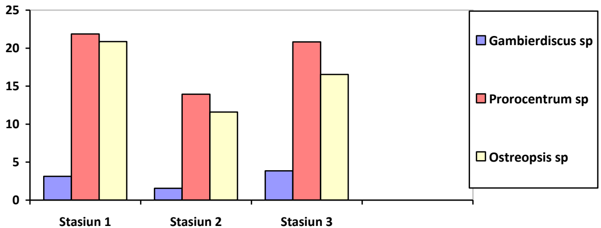
Gambar 1 Kelimpahan dinoflagellata
