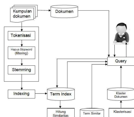
Gambar 3 Arsitektur pencarian dokumen berbasis STC
