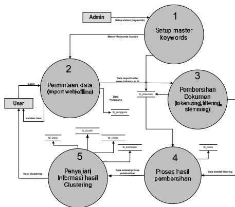
Gambar 4 DFD Level 1
