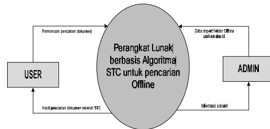
Gambar 1 Diagram Konteks
