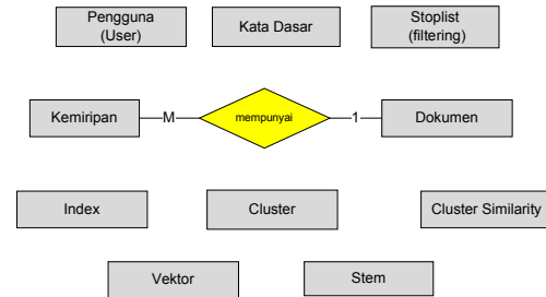
Gambar 5 ERD
