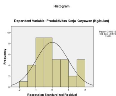
Gambar 2. Grafik Histogram
