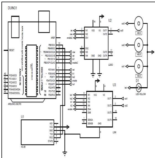
Gambar 3.2 Rangkaian Keseluruhan
