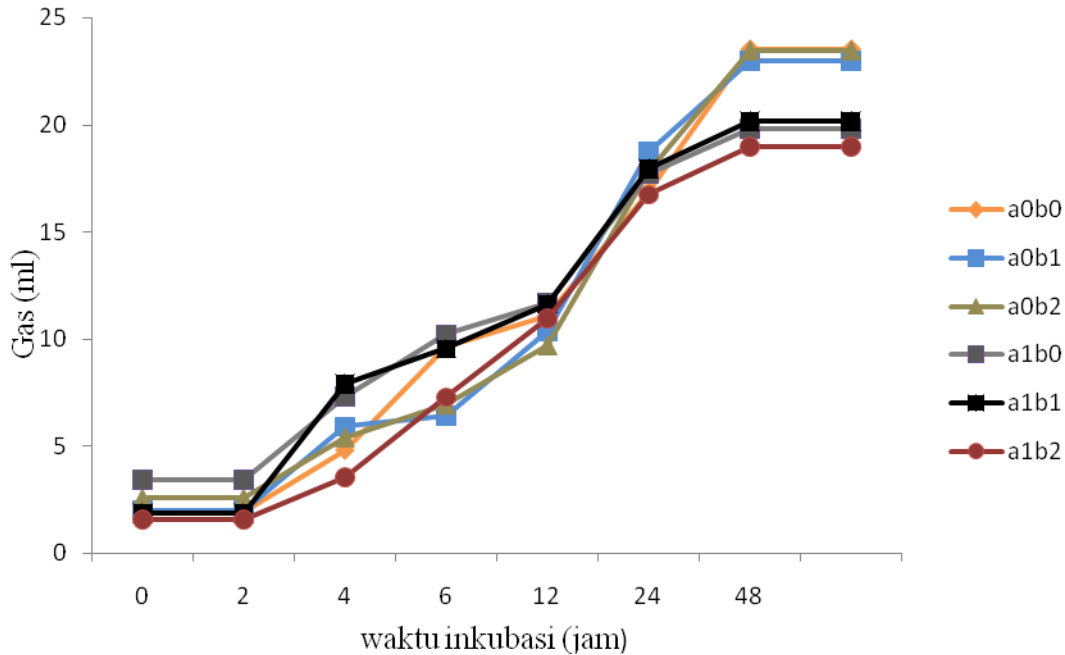
Ilustrasi 4. Kurva Produksi Gas Percobaan selama 48 jam
