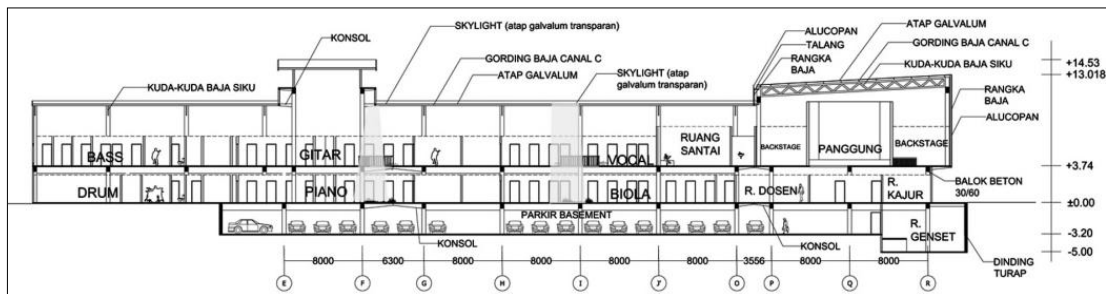
Gambar 2.8. Potongan BB
