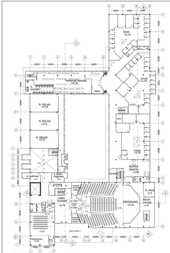
Gambar 2.7. Denah lantai 2
