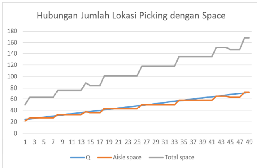
Gambar 7. Grafik Hubungan Jumlah Lokasi Picking dengan Space
