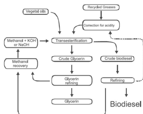
Gambar 3. Proses Produksi Biodiesel (Pinto dkk. , 2005)
