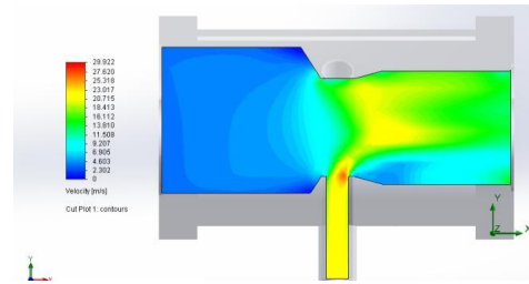
Gambar 16. Hasil simulasi CFD kecepatan aliran campuran udara biogas pada karburetor 3 lubang
