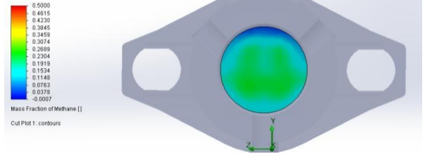
Gambar 15. Hasil simulasi CFD fraksi campuran biogas dan udara pada karburetor 3 lubang (outlet)
