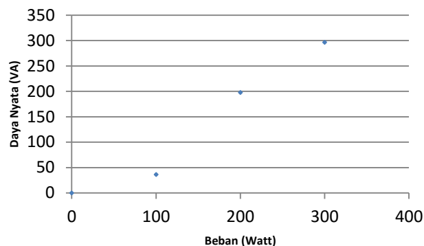
Gambar 4. Grafik kenaikan daya generator set 1 lubang
