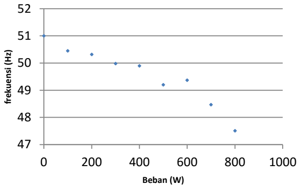
Gambar 9. Frekuensi genset bensin
