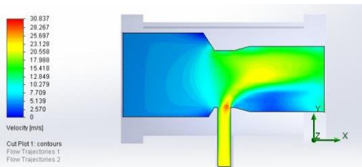
Gambar 14. Hasil simulasi CFD kecepatan aliran campuran udara biogas pada karburetor 2 lubang
