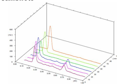
Gambar 8. Profil KLT Tiga Dimensi Sampel EES dan Standar Andrografolid 0,1% b/v
