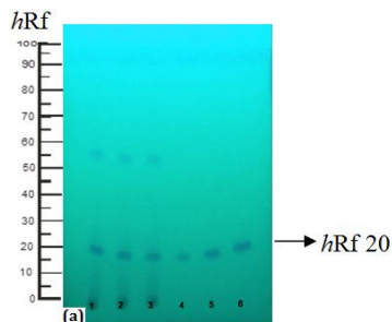
Gambar 3. Kromatogram EES pada UV 254 nm
