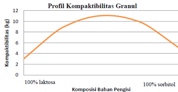
Gambar 7. Profil kompaktilitas granul berdasarkan pendekatan SLD
