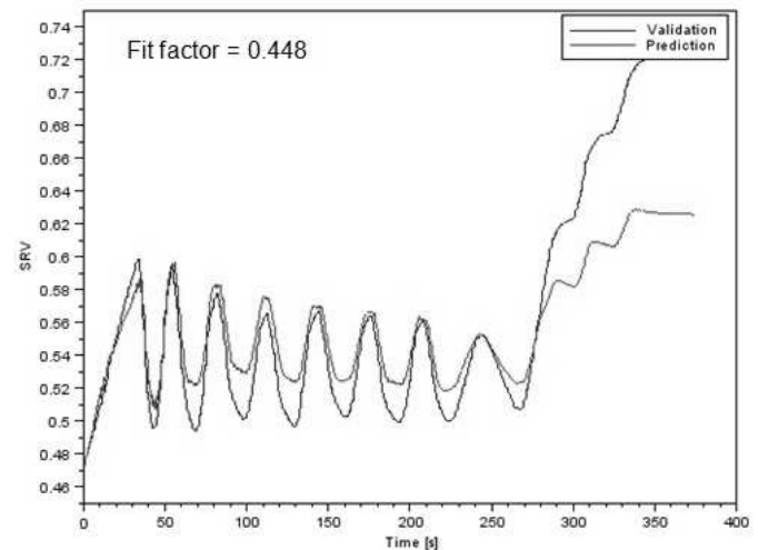
Gambar 6. Hasil identifikasi dengan model ARX
