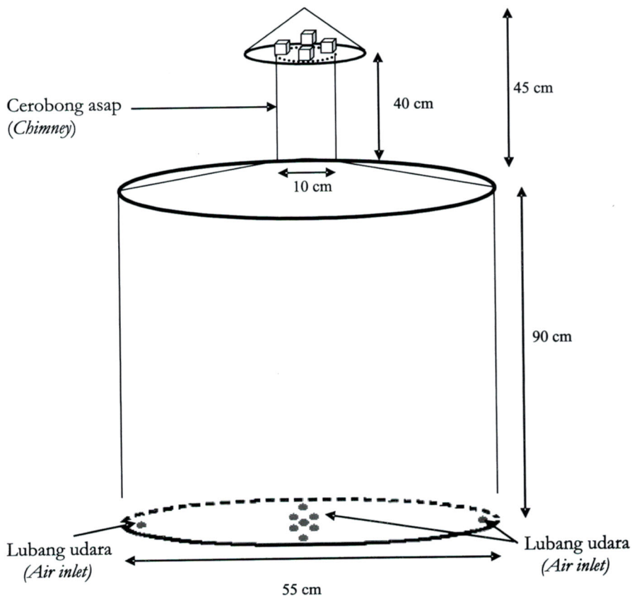
Gambar 1. Tungku arang dari drum oli yang modifikasi Figure 1. Charcoal kiln from modified of drum oil
