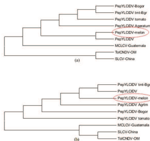
Gambar 7. Dendogram kekerabatan molekuler sampel uji (PepYLCIDV-melon) dan beberapa Begomovirus lain yang telah dipublikasi di database NCBI menggunakan analisis Construct Neighbor-Joining Tree program Mega5: berdasarkan perbedaan sekuen nukleotida dari sebagian sekuen coat protein Begomovirus (a); berdasarkan perbedaan sekuen asam amino dari sebagian sekuen coat protein Begomovirus (b) [PepYLCIDV-Agrtm= AB267838; PepYLCIDV-Bgr= DQ083764; PepYLCIDV tmt-Bgr= DQ083765; PepYLCIDV= AB267834; PepYLCIDV tmt= AB267836; SLCV-China= HM566112; TolCNDV-OM= GU180095; MCLCV-Guatemala= AF325497; sekuen yang dilingkari merupakan sekuen sampel uji (PepYLCIDV-melon)]
