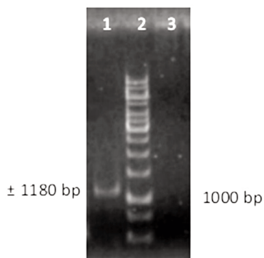
Gambar 4. Hasil deteksi DNA-B Begomovirus pada tanaman melon bergejala daun keriting dengan PCR divisualisasi dengan gel agarose 1% [lajur 1: sampel bergejala daun keriting; lajur 2: marker 1 kb DNA ladder; lajur 3: sampel tidak bergejala daun keriting (kontrol negatif)]
