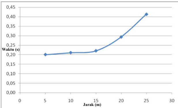
Gambar 22. Grafik pengujian delay gerak robot Fuzzy Sugeno
