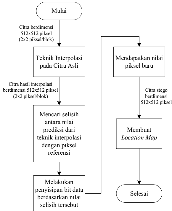
Gambar 2. Proses penyisipan
