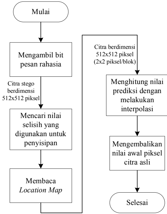
Gambar 5. Proses ekstraksi
