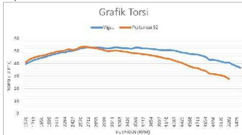
Gambar 4. Grafik Torsi motor berbahan bakar vigas dan pertamax
