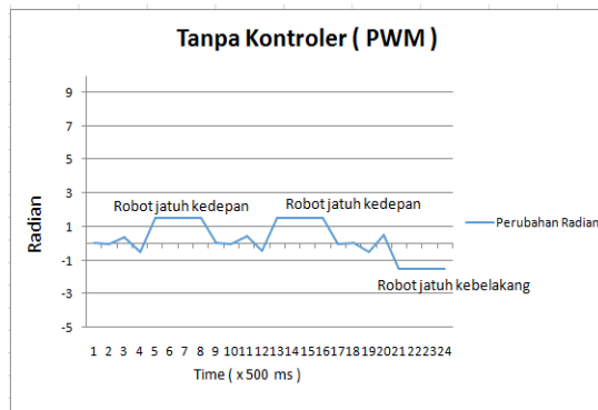
Gambar 4. Pengujian Tanpa Kontroler
