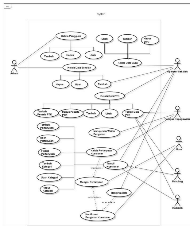
Gambar 2. Use Case Diagram Sistem Evaluasi
