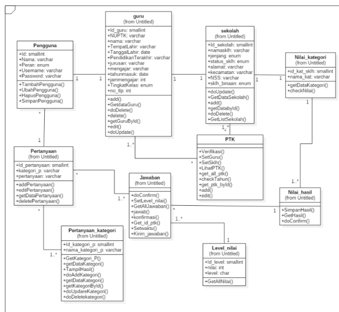
Gambar 3. Class Diagram Sistem Evaluasi
