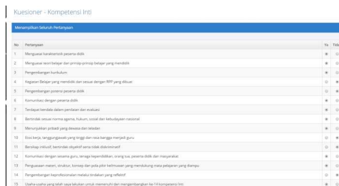
Gambar 5. Pengisian Kuesioner
