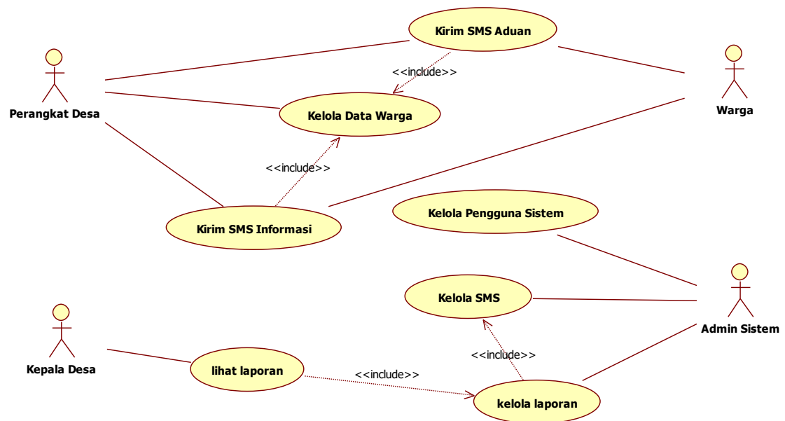
Gambar 2. Use Case Diagram Aplikasi Auto Smart Quick Response Untuk Distribusi Informasi dan Sarana Aduan Masyarakat
