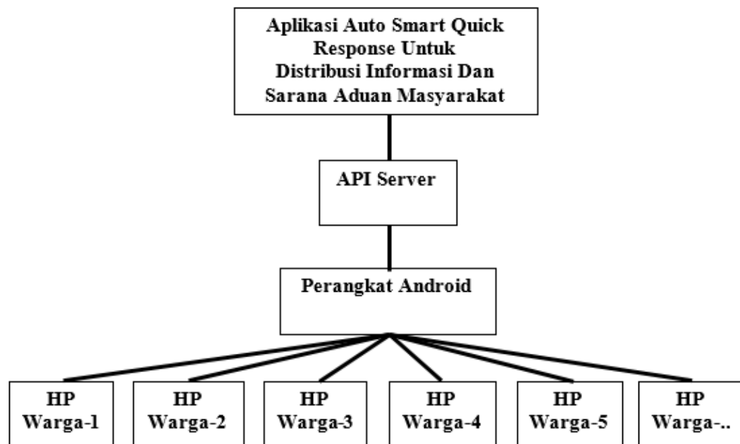
Gambar 1. Arsitektur Aplikasi Auto Smart Quick Response Untuk Distribusi Informasi dan Sarana Aduan Masyarakat
