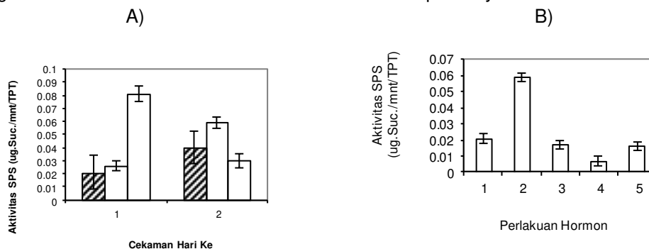
Grafik 3. Pengaruh Aktivitas SPS karena perlakuan : A. Hormon ABA ( □ : Kontrol, ▨ : 10 \mu\text{M} dan □ : 100 \mu\text{M} ) pada hari ke1 dan ke 2. B. 1= Kontrol, 2= ABA , 3= BA , 4= JA dan 5= IAA masing-masing dengan konsentrasi 10 \mu\text{M}
