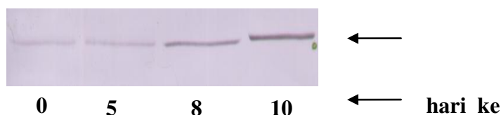
Gambar 1. Analisis Western Blot protein SPS-1 Kultivar M442-51 karena perlakuan Cekaman Kekeringan. Protein dipisahkan menggunakan elektroforesis SDS-PAGE 12,5 %, masing-masing kolom berisi 30 \mu g
