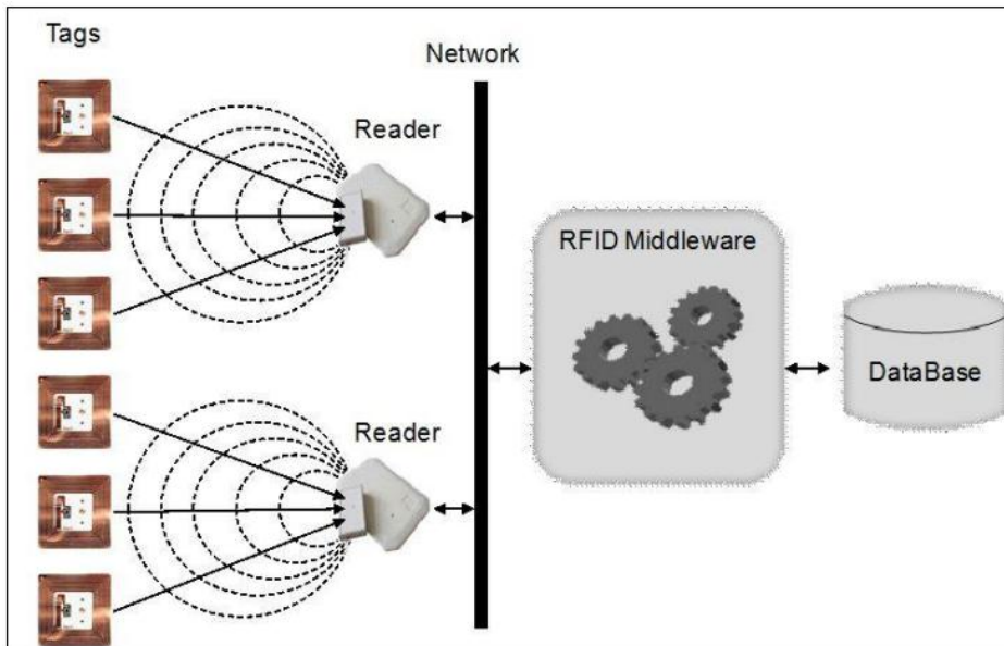
Gambar 7. Blok Diagram Sistem
