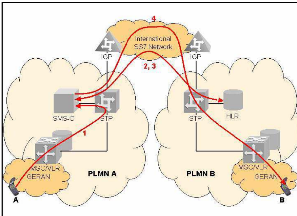
Gambar 1. Susunan Jaringan dan Aliran Message
