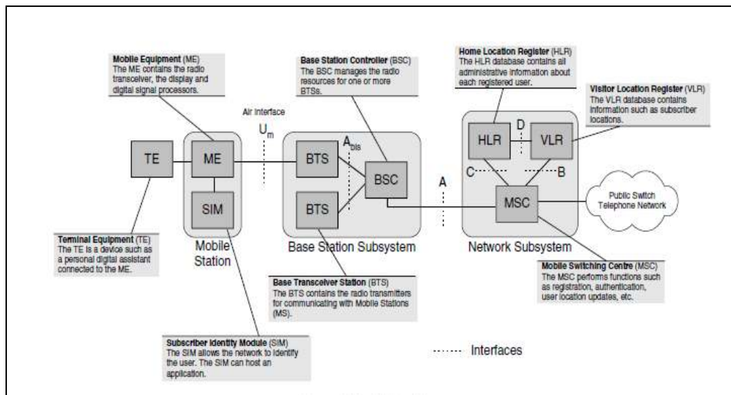
Gambar 3. Arsitektur GSM
