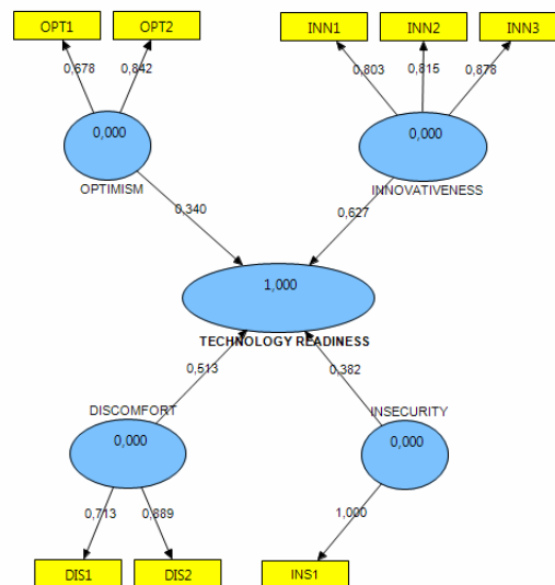
Gambar 3. Path diagram setelah dimodifikasi
