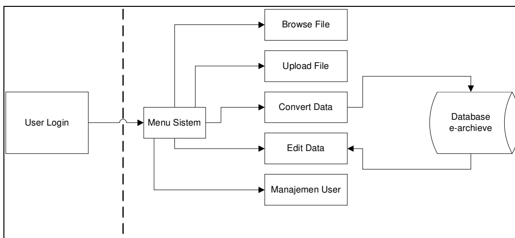
Gambar 4.1 Arsitektur Aplikasi
