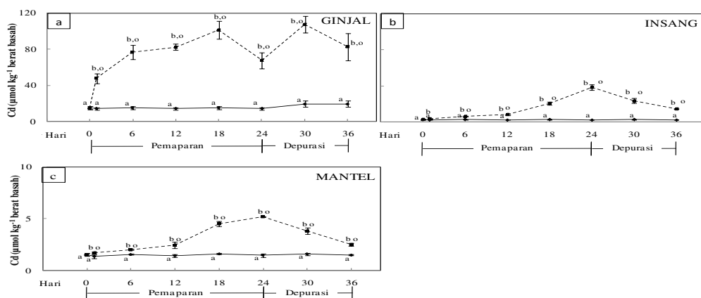
Gambar 1. Bioakumulasi Cd pada organ Elongaria orientalis : (a) ginjal; (b) insang; (c) mantel (Ket: \diamond = kontrol; \blacksquare = perlakuan). Beda nyata terhadap kontrol hari ke-0 ditandai dengan simbol ^{\circ} ( p < 0,05 ). Huruf yang sama menunjukkan pemaparan tidak berbeda nyata terhadap kontrol pada masing-masing perlakuan.
