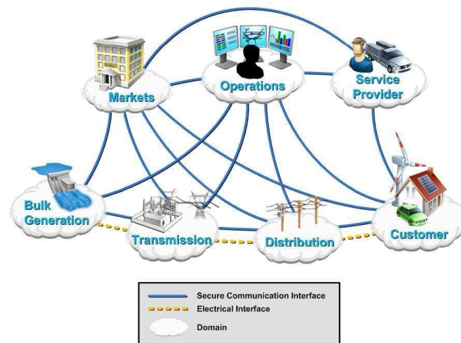
Gambar 4.3 Konsep SMART GRID secara keseluruhan
