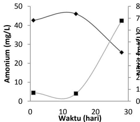
Gambar 2. Perubahan Amonium (♦) dan Nitrit (■) pada Proses Anammox di Air Lindi
