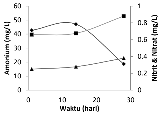
Gambar 1 Perubahan Amonium (♦), Nitrit (■), dan Nitrat (▲) pada Proses Nitrifikasi di Air Lindi
