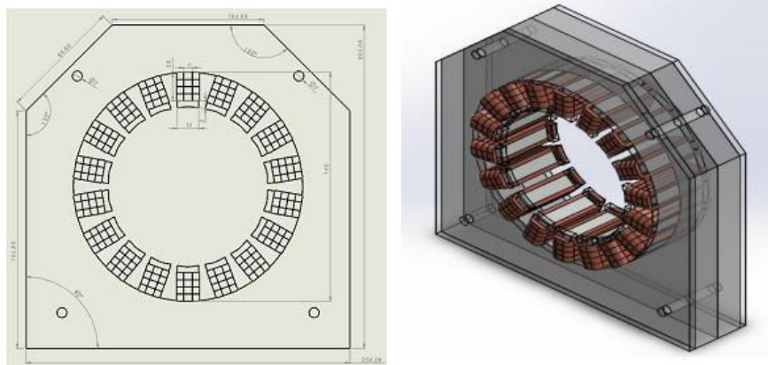
Gambar 3. Sketsa 2 dimensi dan 3 dimensi dari stator
